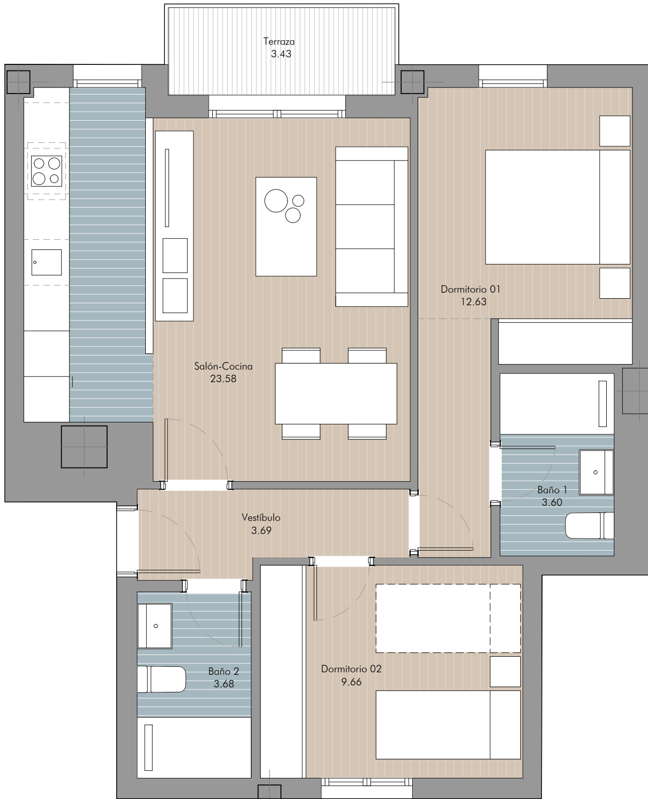
Planta Segunda
